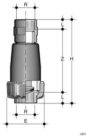
Донный клапан VZFV ПВХ с резьбовыми окончаниями, EPDM, FIP R1" (DN25)
