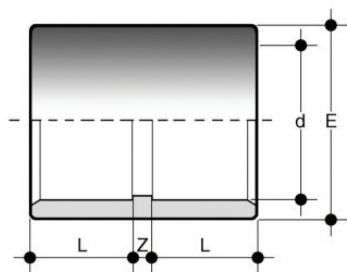
Соединительная муфта ХПВХ d75 PN16
