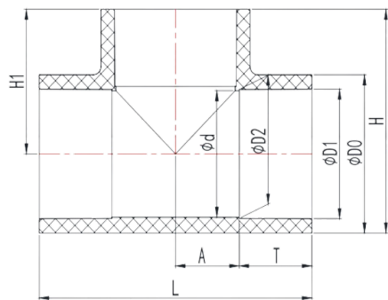
Тройник равнопроходной клеевой 90° ПВХ IPS d110
