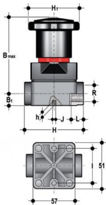
Компактный мембранный клапан CM ПВДФ с резьбовыми окончаниями R1/2" (DN15)
