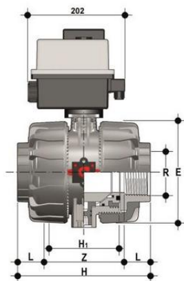
Шаровой кран VKD ПВХ с эл.приводом 24V AC/DC, резьбовые окончания, EPDM, FIP R2 1/2" (DN65)
