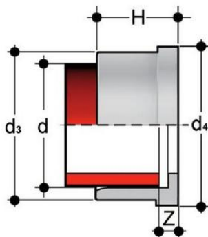
Муфтовое окончание ПВДФ d32 SDR21 PN16
