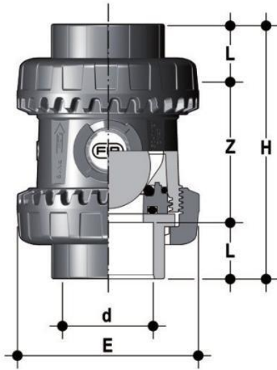
Шаровой обратный клапан SXEIV ПВХ; с муфтовыми окончаниям, ФKM, FIP d40 (DN32)
