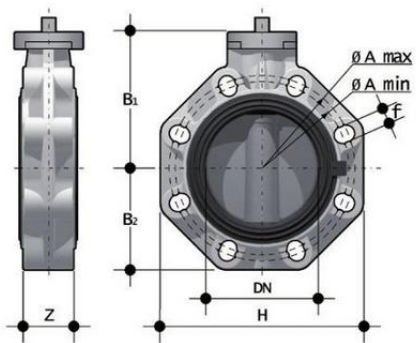
Дисковый затвор ПВХ ФКОАВФМ со свободным штоком, EPDM, FIP d12" (DN300)
