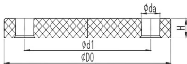
Глухой фланец ПВХ IPS d63
