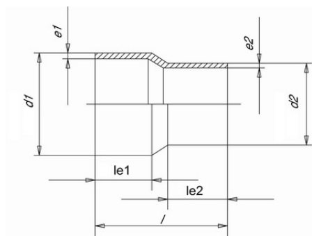
Муфта редукционная ПВДФ (Simona) 50x32 SDR21 PN16
