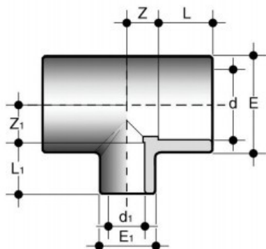
Тройник редукционный ПВХ FIP 90x75
