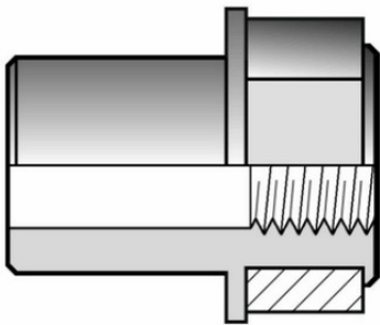
Адаптер с внутренней резьбой PP-H FIP 63x2 SDR11 PN6
