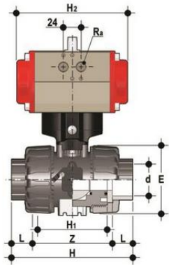
Шаровой кран VKD ПВХ с пневмоприводом НЗ с резьбовыми окончаниями, EPDM, FIP R3/8" (DN10)
