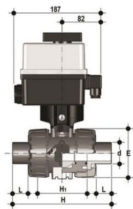
Шаровой кран VKD ХПВХ с эл.приводом 24V AC/DC, втулочные окончания d40 (DN32)
