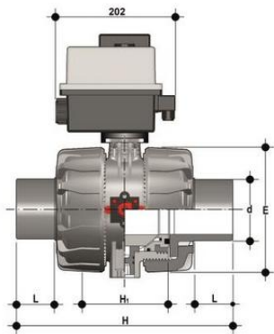
Шаровой кран VKD ПВДФ с эл.приводом 90-240V, втулочные окончания d90 (DN80)
