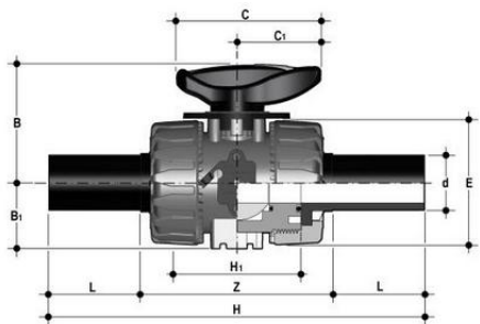
Шаровой кран для регулирования потока VKR с партрубками из ПЭ (уплотнение EPDM) PP-H d40 (DN32)
