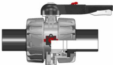
Шаровой кран промышленного применения VKD с патрубками из ПЭ (CVDE) (уплотнение FKM) PP-H d75 (DN65)
