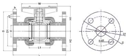
Кран шаровой промышленного применения, фланцевые окончания, FKM, IPS d50
