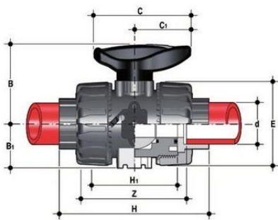
Шаровой кран VKD ПВДФ с муфтовыми окончаниями d25 (DN20)
