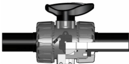
Шаровой кран ПВХ промышленного применения VKD с патрубками из ПЭ (CVDE), FKM, FIP d32 (DN25)
