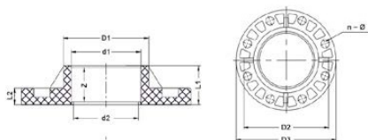
Жесткий фланец ХПВХ IPS (Model B) d355 PN10
