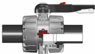
Шаровой кран промышленного применения VKD с патрубками из ПЭ (CVDE) (уплотнение EPDM) PP-H d75 (DN65)
