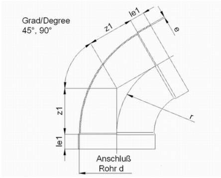
Изгиб 90° PPs d710
