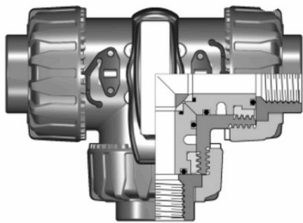
3-х ходовой шаровой кран ТКД ХПВХ с резьбовыми окончаниями, L-шар R2" (DN50)
