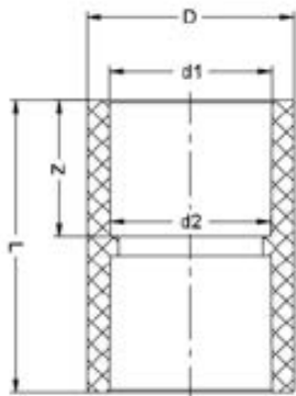
Муфта соединительная ХПВХ IPS (Model B) d315 PN10
