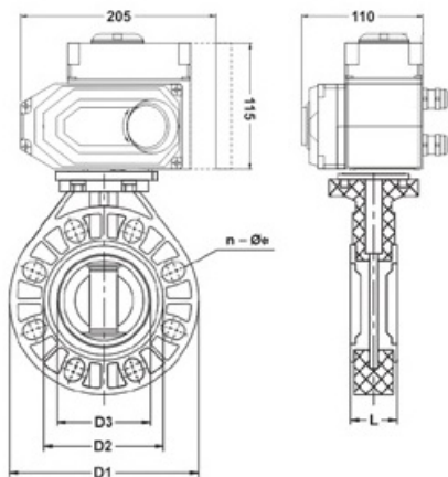
Дисковый затвор IFK ПВДФ с электрическим приводом 220V AC, FKM, IPS d90 (DN80)
