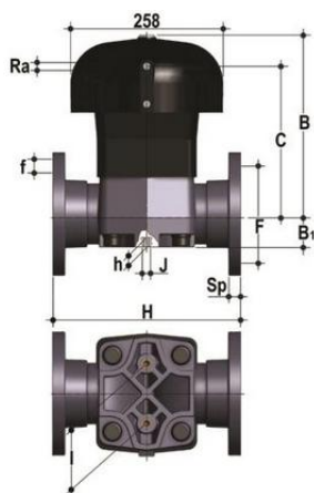
Мембранный клапан VMOC ХПВХ с втулочными окончаниями d110 (DN90)
