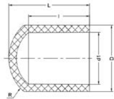
Заглушка ПВДФ для стыковой сварки d25 PN 16
