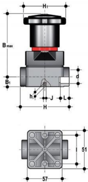
Компактный мембранный клапан CM ПВХФ с муфтовыми окончаниями d20 (DN15)
