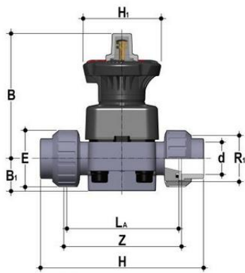
Мембранный клапан DK/L ПВДФ с муфтовыми окончаниями d32 (DN25)
