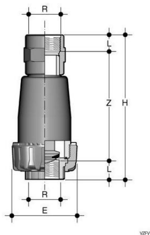
Донный клапан VZFV ПВХ с резьбовыми окончаниями, EPDM, FIP R1½" (DN40)
