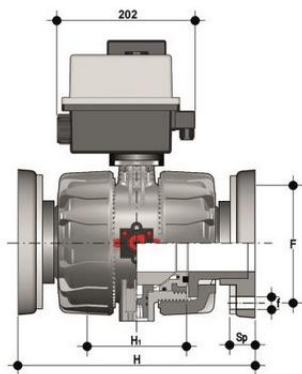
Шаровой кран VKD с эл.приводом 24V AC/DC, фланцевые окончания, DN65-100 (уплотнение FKM) PP-H d110 (DN100)
