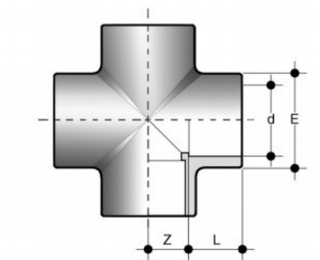
Крестовина клеевая ПВХ FIP d50
