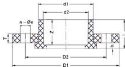
Фланец свободный с буртом ХПВХ IPS (Model B) - комплект d400 PN10
