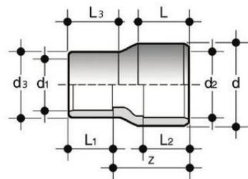
Втулка редукционная ПВХ FIP (четырёхразмерная) 90x75x75x63
