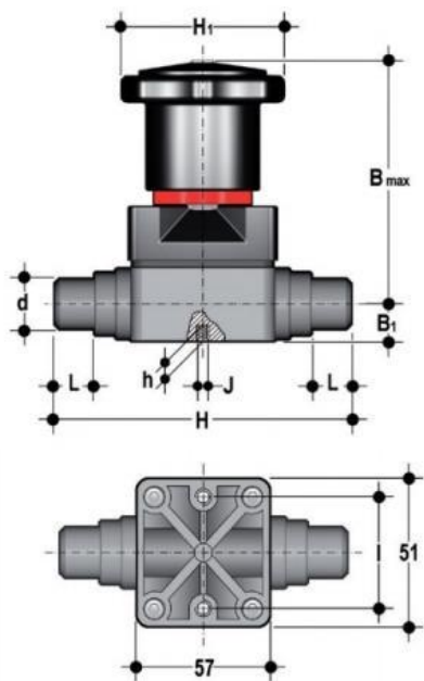
Компактный мембранный клапан CM с втулочными окончаниями (уплотнение EPDM / мембрана EPDM) PP-H d20 (DN15)
