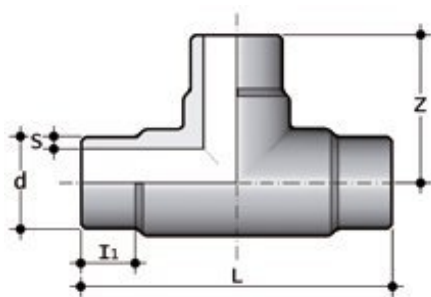
Тройник равнопроходной для стыковой сварки PP-H FIP d110 SDR17.6 PN10
