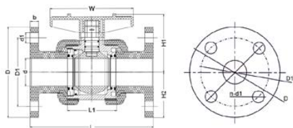
Кран шаровой промышленного применения, фланцевые окончания, EPDM, IPS d32
