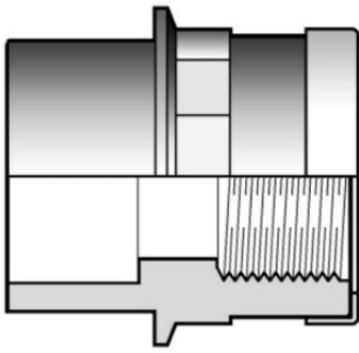
Двойной муфтовый адаптер с ВР и усиливающим кольцом ПВХ FIP 25x20x1/2
