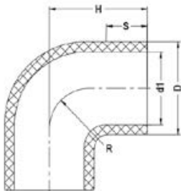
Отвод ПВДФ 90° d90 PN 16
