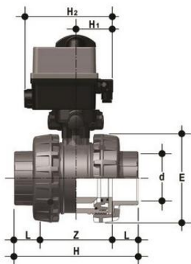
Шаровой кран VXE ПВХ с пневмоприводом, EPDM, FIP d90 (DN80)
