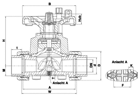
Мембранный клапан ПВХ с муфтовыми окончаниями, FKM, Praher Plastics d20 (DN15)
