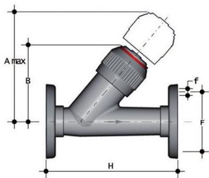
Угловой обратный клапан VROV ПВХ с фланцевыми окончаниями, EPDM, FIP d50 (DN40)
