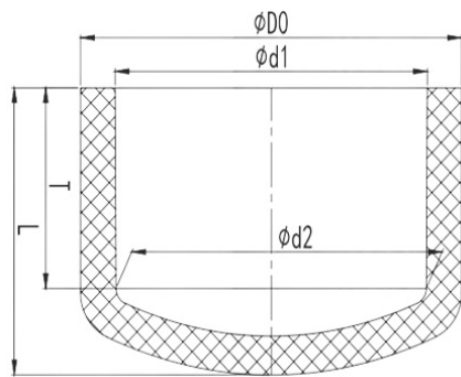
Заглушка клеевая ПВХ IPS d315
