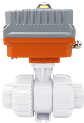
Шаровой кран IVKD ПВДФ с эл.приводом 220V AC, муфтовые окончания, EPDM, IPS d75 (DN65)
