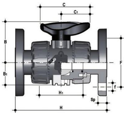
Шаровой кран промышленного применения VKD с фланцевыми окочаниями (уплотнение FKM) PP-H d25 (DN20)
