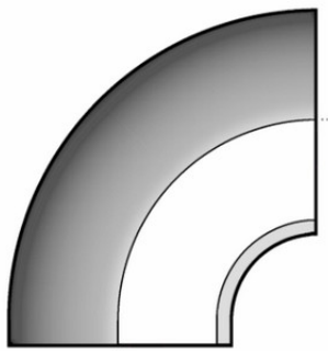
Отвод 90° для стыковой сварки PP-H FIP (PN 10) d280 SDR11 PN10
