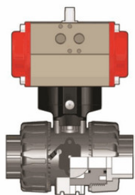
Шаровой кран VKD ПВХ с пневмоприводом ДвД с резьбовыми окончаниями, EPDM, FIP R3/8" (DN10)
