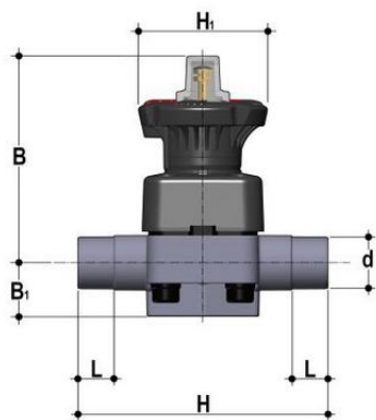
Мембранный клапан DKLDV ПВХ с муфтовыми окончаниями, PTFE, FIP d50 (DN40)
