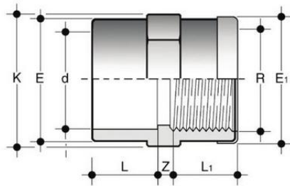
Переходная муфта с усиливающим кольцом ХПВХ 50x1 1/2" PN16
